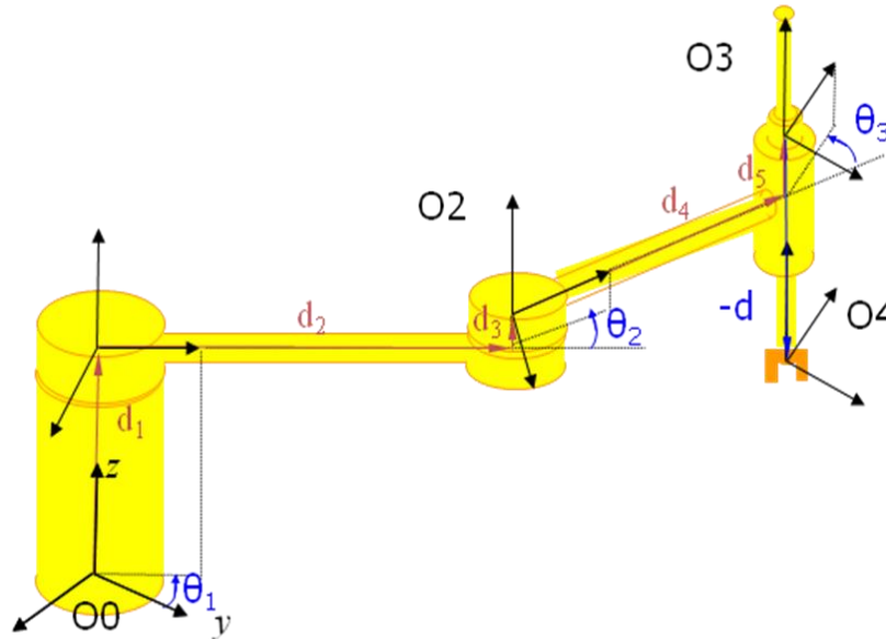
Figur 3. En robottillämpning av koordinattransformationer
