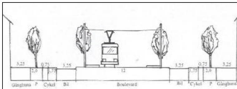
Sektion Hagebygatan.
